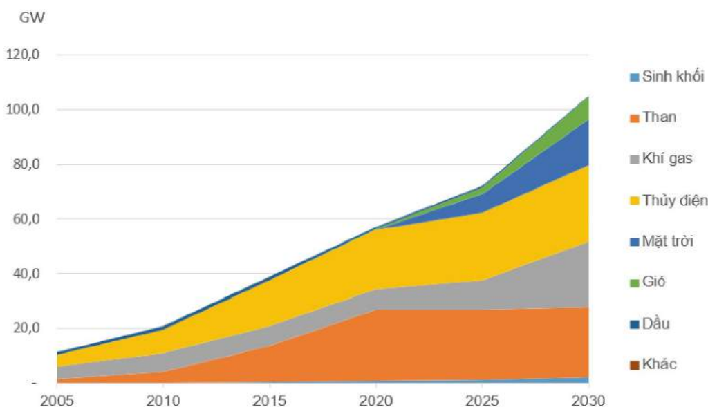
Hình 23: Phát triển công suất tương lai theo kịch bản EE&RE
