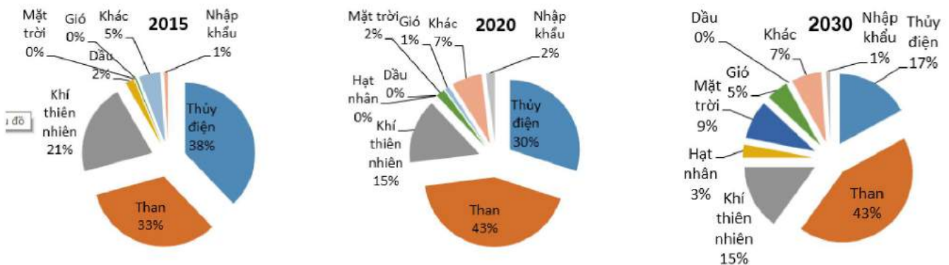
Hình 1: Tỷ lệ công suất các nguồn điện theo dạng nhiên liệu
