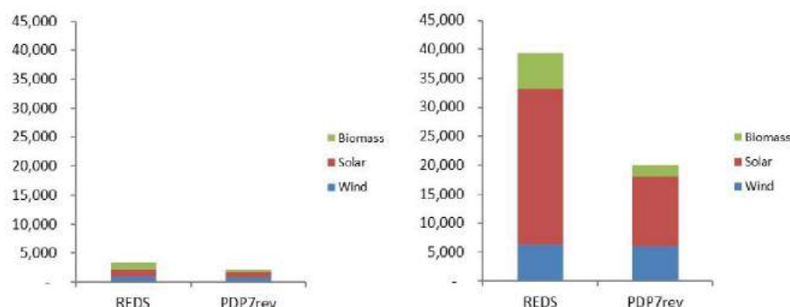
Hình 2 : Các mục tiêu về NLTT (MW) trong QHĐ VII điều chỉnh và REDS năm 2020 và 2030
