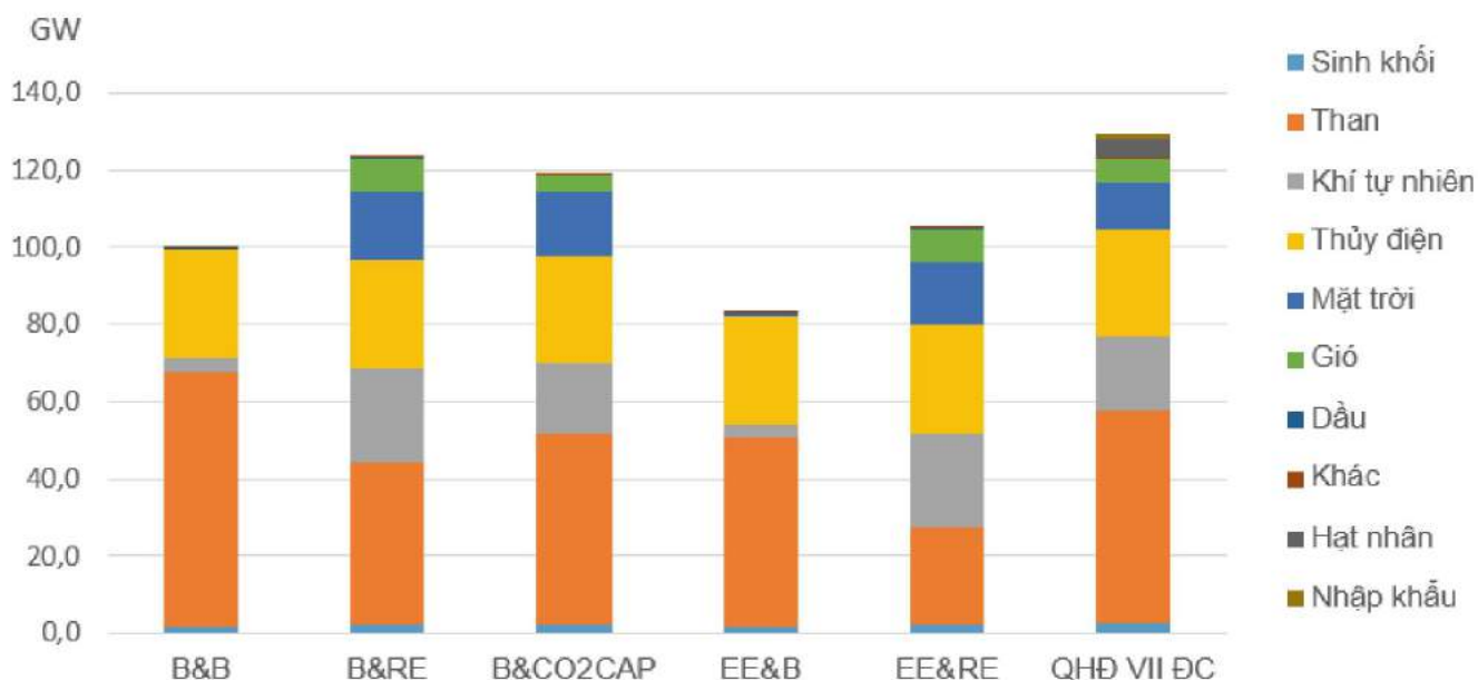
Hình 24: Công suất của các kịch bản vào năm 2030
