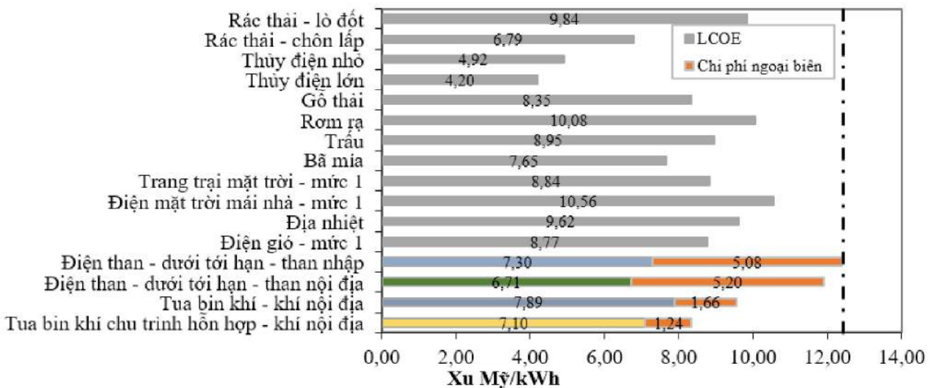
Hình 18: Chi phí sản xuất điện quy dẫn có xem xét đến chi phí ngoại biên của các công nghệ phát điện năm 2017
