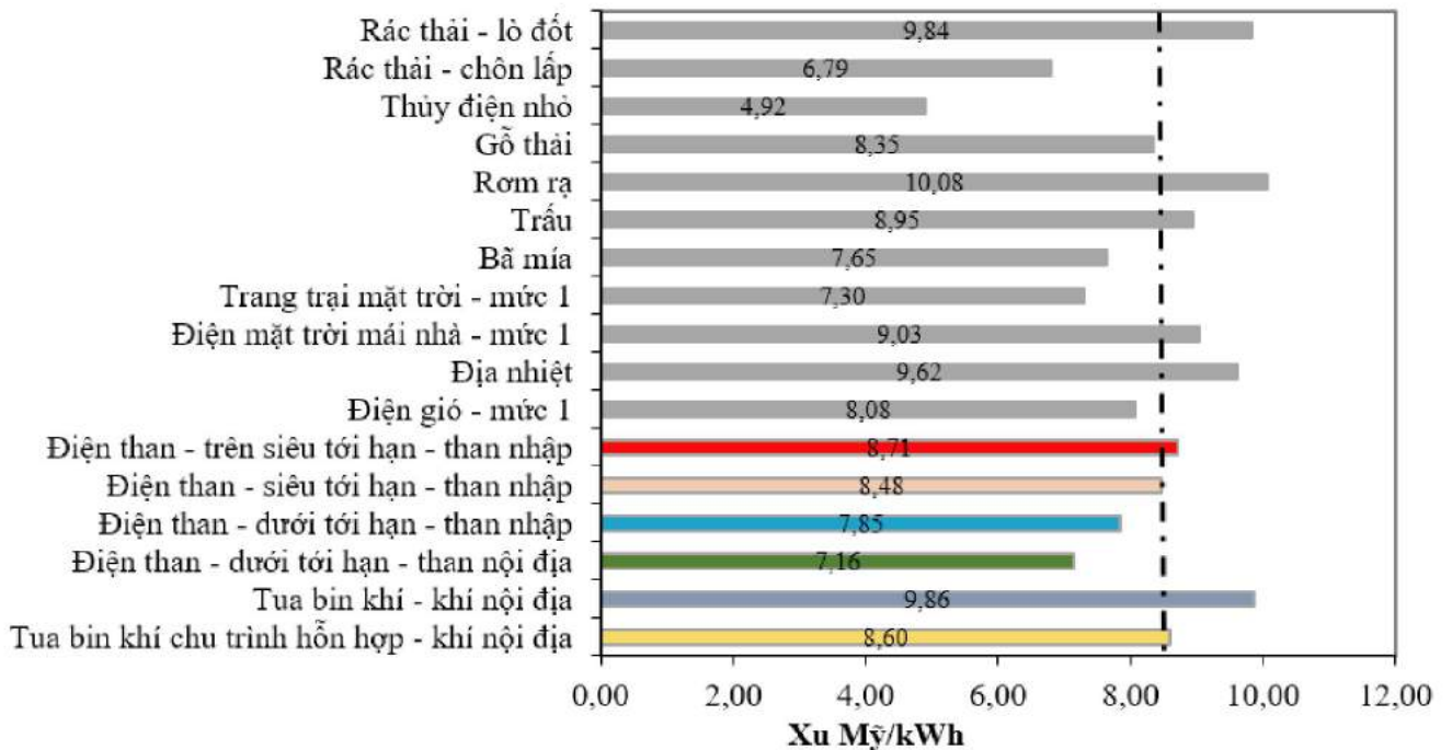
Hình 17: Chi phí sản xuất điện quy dẫn của các công nghệ phát điện được đầu tư năm 2030
