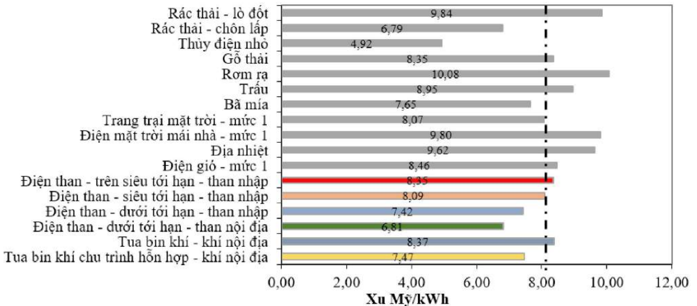
Hình 15: Chi phí sản xuất điện quy dẫn của các công nghệ phát điện được đầu tư năm 2020
