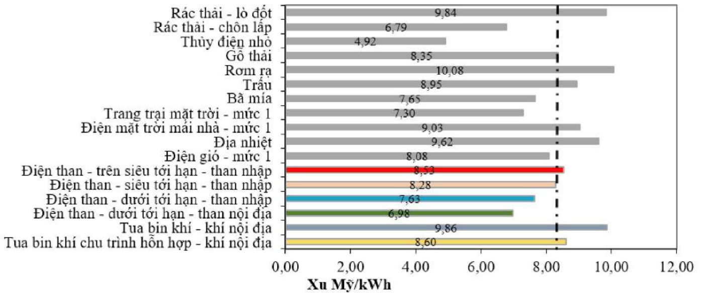
Hình 16: Chi phí sản xuất điện quy dẫn của các công nghệ phát điện được đầu tư năm 2025
