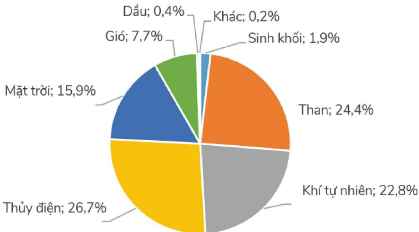
Cơ cấu công suất nguồn điện đề xuất đến 2030
