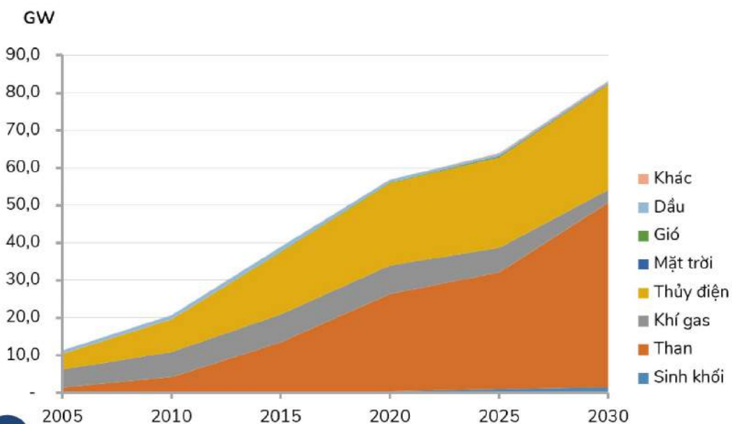
Hình 22: Phát triển công suất tương lai theo kịch bản EE&B
