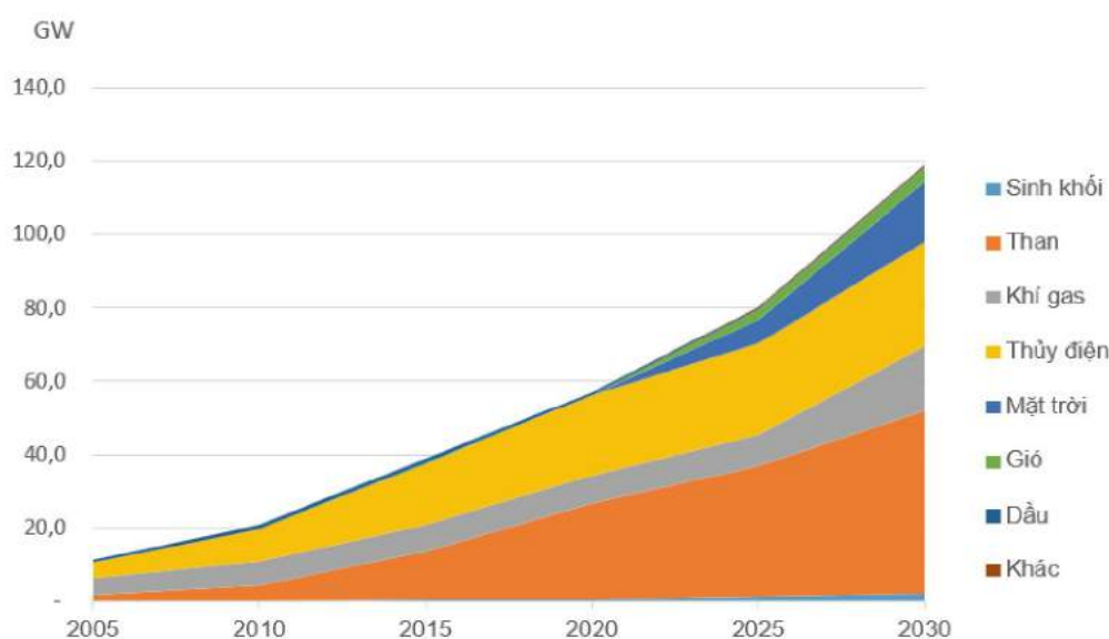
Hình 21: Phát triển công suất tương lai theo kịch bản kiểm soát phát thải
